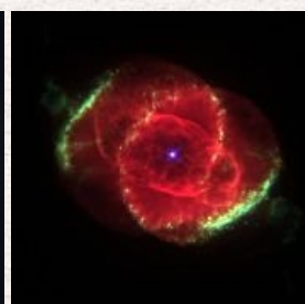
NGC 6543
